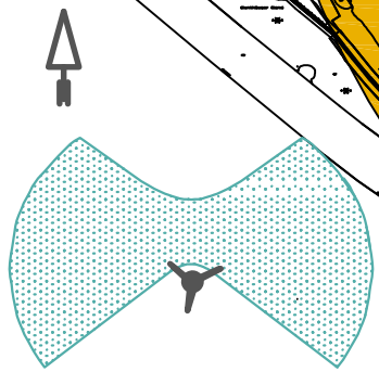
Theoretischer Schattenwurf einer Windkraftanlage
